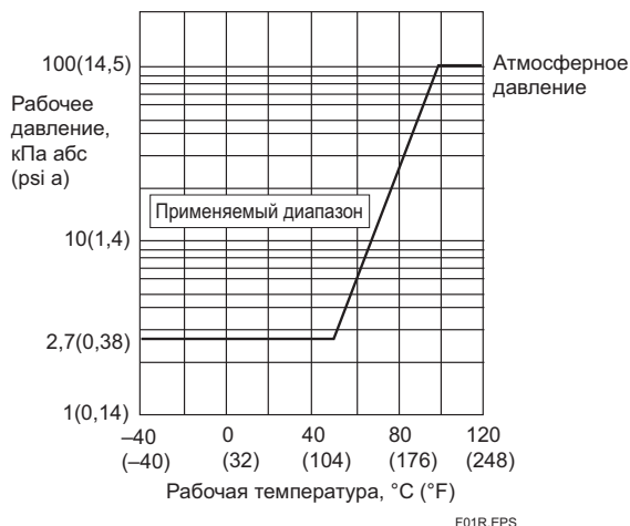
Рис. 1. Температура процесса и рабочее давление
